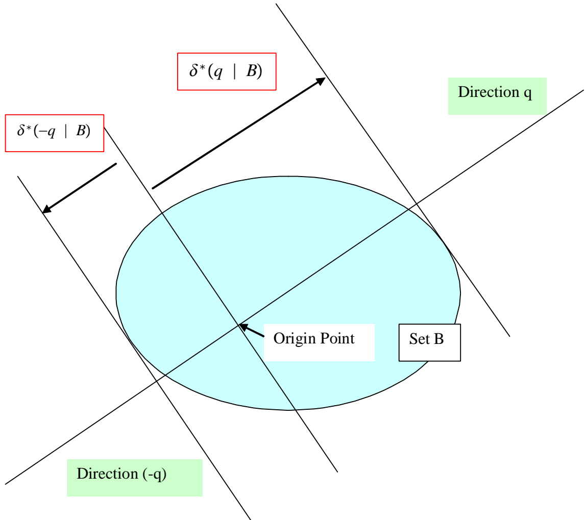
Figure 2: La fonction support d'un ensemble convexe
